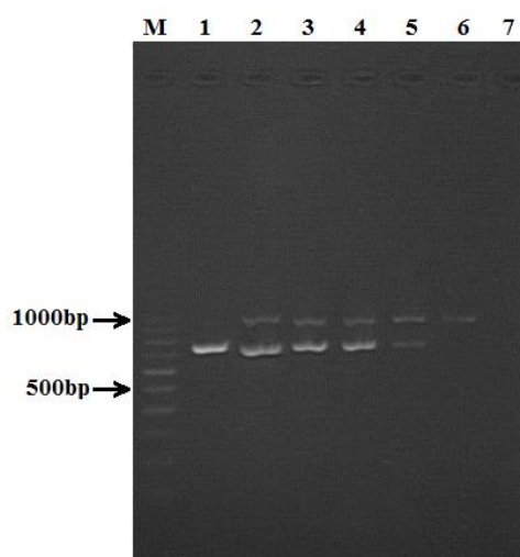
Figure 4. Resolution of mixtures of Tetranychus species. Lane M: DNA size marker; Lane 1: 5 T. urticae ; Lane 2: 4 T. urticae +1 T. turkestanii ; Lane 3: 3 T. urticae +2 T. turkestanii ; Lane 4: 2 T. urticae +3 T. turkestanii ; Lane 5: 1 T. urticae +4 T. turkestanii ; Lane 6: 5 T. turkestanii , Lane 7: C.
