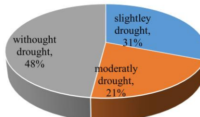
SDI Index(2016-2044)
