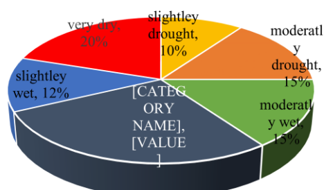
SWSI Index(2016-2044)
