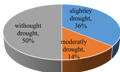
SDI Index(1987-2015)
